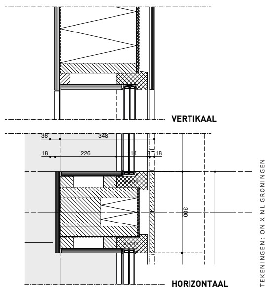
Wegdetailering van het kozijn in houten kolom.
